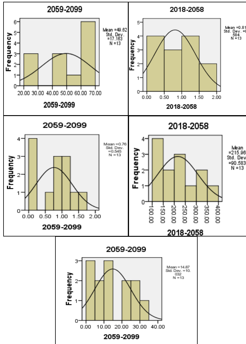
ادامه شکل (۴). روند معنی داری و نزولی و صعودی پارامترهای اقلیمی موثر در شاخص تریجونگ (۱۹۸۷-۲۰۹۹) منبع: (۲۰۹۹) (نگارنده)
