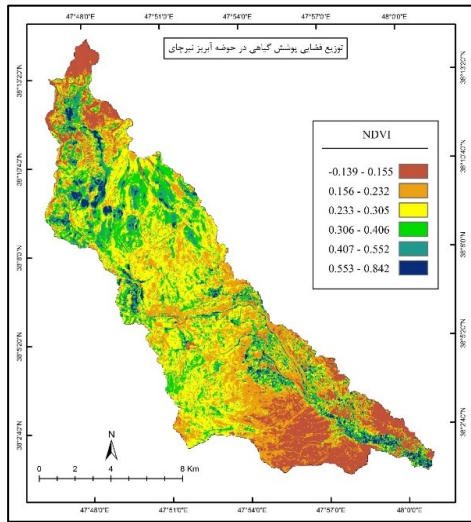
شکل (۴). پوشش گیاهی (NDVI) حوضه نیرچای
