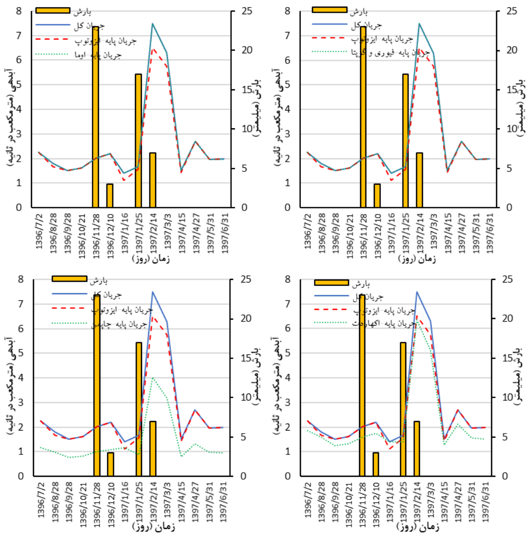
شکل (۳). مقایسه الگوهای مختلف روش RDF با مقادیر ایزوتوپی اکسیژن ۱۸- چشمه کهمان.
