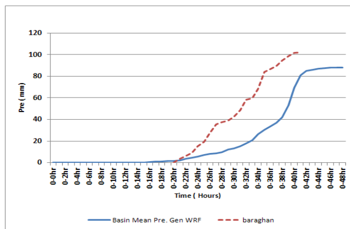
شکل (۳). مقایسه تغییرات الگوی زمانی بارش ایستگاه برغان و مدل عددی WRF (کل حوضه) بازه زمانی ۱۴ و ۱۵ آذر ۱۳۸۲
