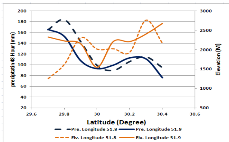
شکل (۱۲). تغییرات بارش با ارتفاع و عرض جغرافیایی در طول جغرافیایی 51/8 و 51/9 درجه توفان ۴۸ ساعته ۱۴ تا ۱۵ آذر ۱۳۸۲ در محدوده حوضه سد پارسیان
