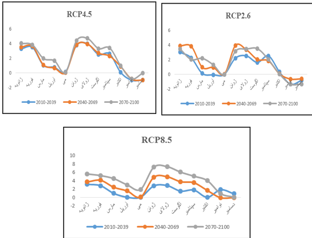
اشکال (۷ تا ۹). تغییرات میانگین دمای ایستگاه اهر طی دوره‌های مختلف مورد مطالعه تحت سناریوهای RCP2.6، RCP8.5 و RCP4.5
