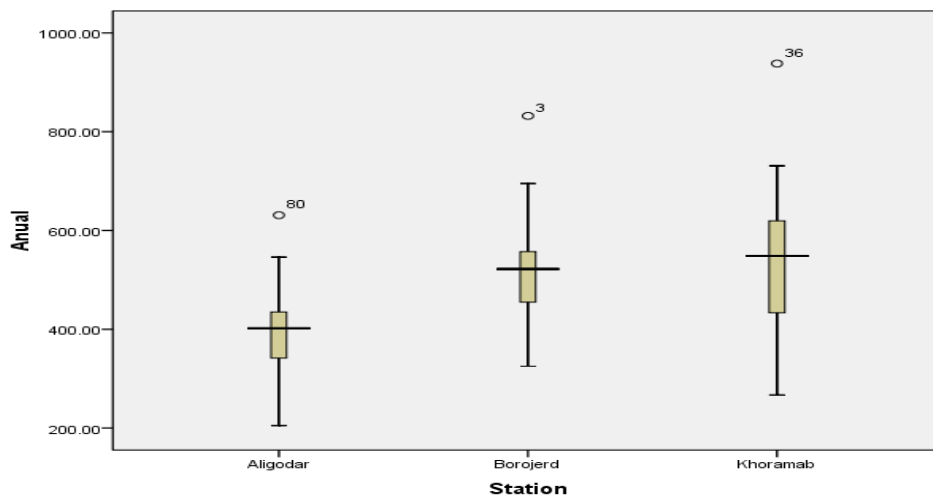
شکل (۲). توزیع بارش در ۳ ایستگاه خرم آباد، بروجرد و الیگودرز
