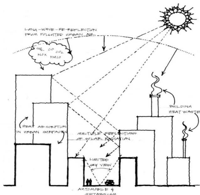
شکل (۱). تأثیر ضریب دید آسمان در تابش ورودی و خروجی چتر شهری (Emmanuel, ۲۰۰۵)
