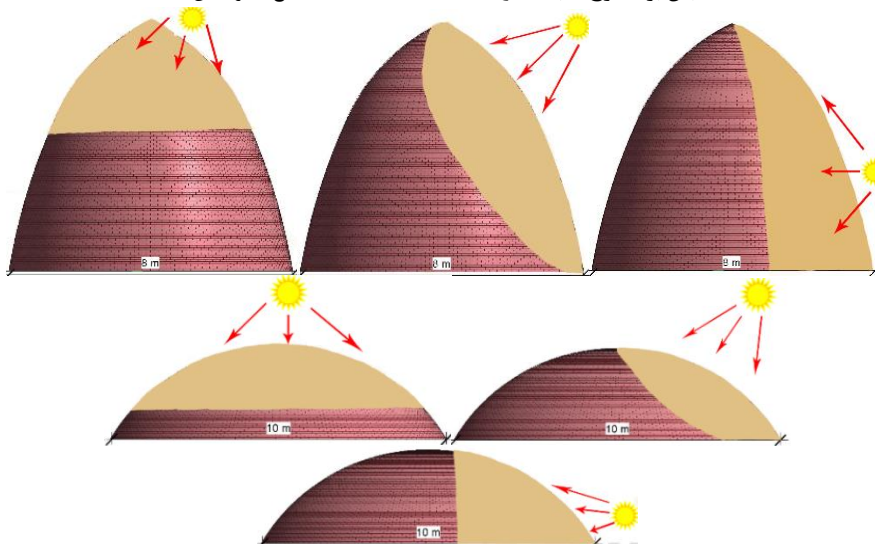
شکل (۱۰). از سمت بالا تصاویر گرافیکی میزان دریافت تابش بر سطوح گنبد خیز بلند در سه بازه‌ی زمانی روز (۱۳، ۱۴، ۱۶). از سمت پایین تصاویر گرافیکی میزان برخورد تابش خورشید بر سطوح گنبد آبناهارهای خیز کم در سه بازه‌ی زمانی روز (۱۳، ۱۴، ۱۶). منبع: نگارندگان.
