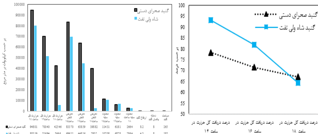
شکل (۷). نمودار از سمت چپ مربوط به میزان دریافت حرارت در معرض تابش، در محدوده سایه و حرارت کل گنبد آبنا‌رهای دهانه ثابت شهر یزد در گرم‌ترین روز سال در ساعات ۱۴، ۱۶، ۱۸ بعدازظهر نمودار از راست درصد میزان دریافت تابش خورشید بر سطوح گنبدهای با دهانه ثابت یزد در ساعات ۱۴، ۱۶، ۱۸ بعدازظهر، منبع: نگارندگان.
