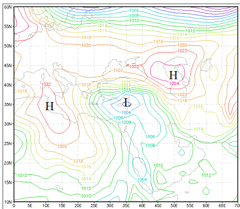
شکل (۸). میانگین فشار تراز دریا ۳۱ مارس ۲۰۱۹
