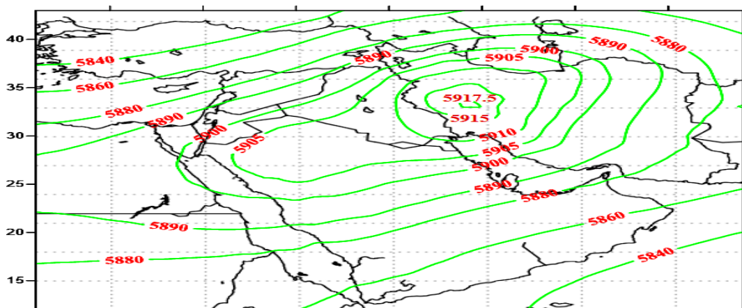
شکل (۱۲). آرایش الگوی متوسط ارتفاع ژئوپتانسیل تراز ۵۰۰ hp در الگوی سوم (میانگین ۱۸۱ روزه)
