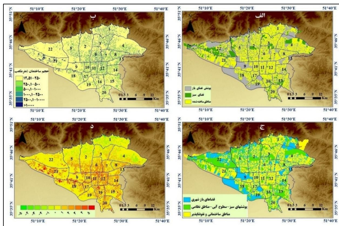
شکل (۴). نقش متغیرهای محیطی انسان ساخت در ارتباط با جزیره گرمای شهری، الف: پوشش زمینی، ب: حجم ساختمان، ج: مجاورت با فضاها، د: بار گرمایی
