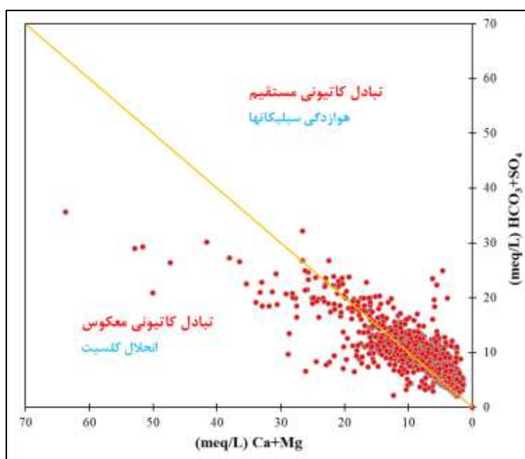
شکل (۷). موقعیت نمونه‌های مورد مطالعه در نمودار دو متغیره \text{Ca}+\text{Mg} نسبت به \text{SO}_4+\text{HCO}_3
