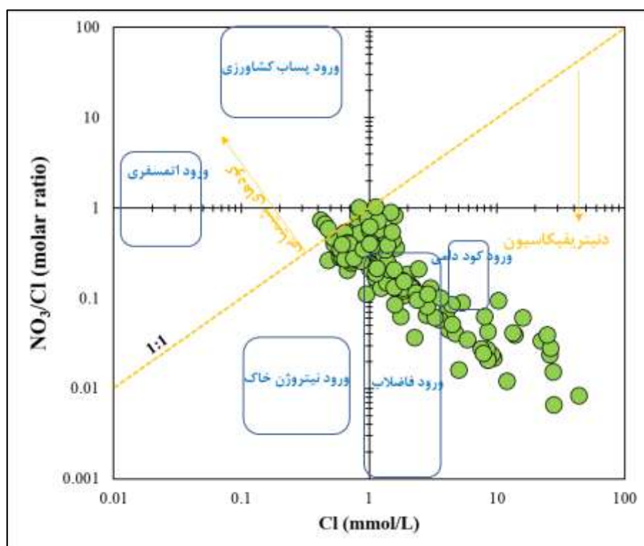
شکل (۱۲). شناسایی منابع احتمالی نترات در آب زیرزمینی بر اساس نسبت \text{NO}_3/\text{Cl} در مقابل \text{Cl}
