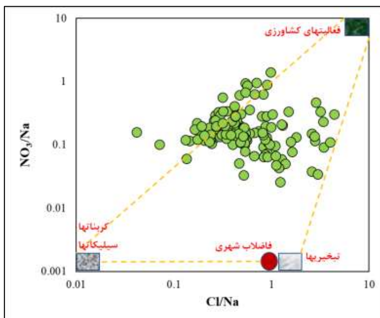
شکل (۱۰). موقعیت نمونه‌های آب زیرزمینی بر روی نمودار \text{NO}_3/\text{Na} در مقابل \text{Cl/Na}
