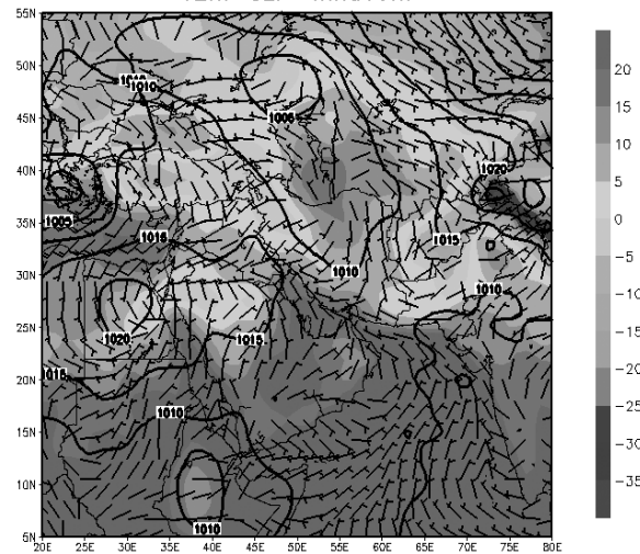
شکل ۱۹: فشار سطح دریا (خطوط هم‌مقدار بر حسب هکتوپاسکال)، دمای ۲ متری (بخش‌های رنگی شده بر حسب درجه‌ی سلسیوس) و باد ۱۰ متری (بر حسب متر بر ثانیه)، برای ساعت ۱۲ گرینویچ روز ۱۳ دسامبر ۲۰۱۰.
