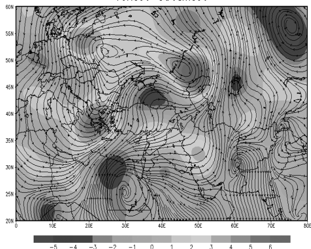
شکل ۲۰: میدان تاوایی نسبی (مقادیر رنگی شده برحسب عکس ثانیه) و جریان تراز ۸۵۰ هکتوپاسکالی (خطوط پیوسته) برای ساعت ۱۲ گرینویچ روز ۱۳ دسامبر ۲۰۱۰.
