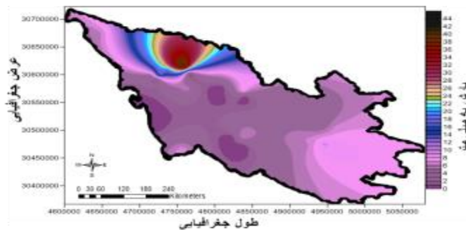
شکل ۱۴: نقشه پهنه بندی بارش سنگین در روز ۲۹ نوامبر ۱۹۹۶
