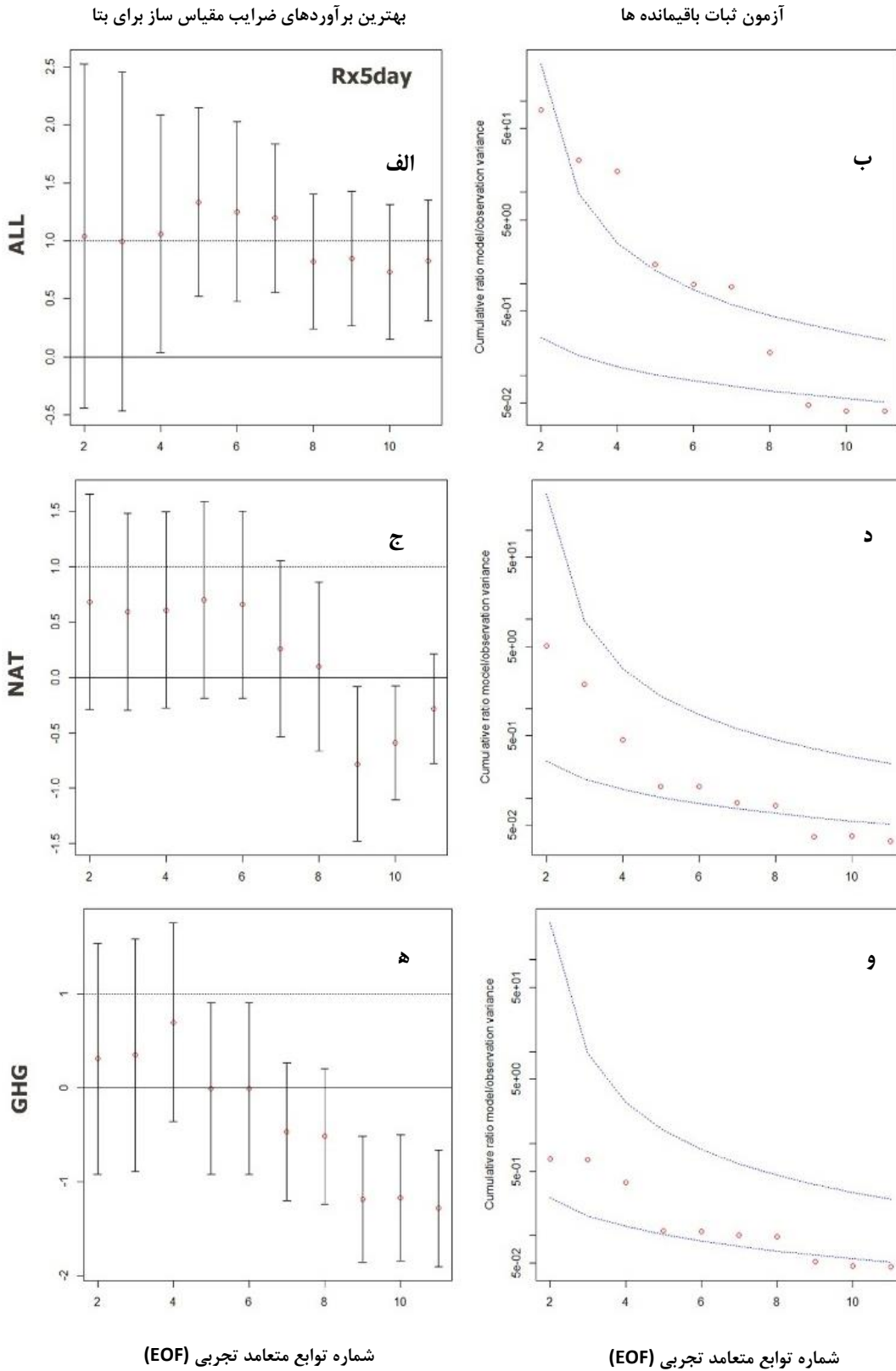
شماره توابع متعامد تجربی (EOF) شماره توابع متعامد تجربی (EOF) شکل ۲: بهترین ضرایب مقیاس ساز برای سیگنال‌های ALL, NAT, GHG مربوط به Rx5day (کادر سمت چپ) و نتایج آزمون ثبات باقیمانده‌ها (کادر سمت راست)
