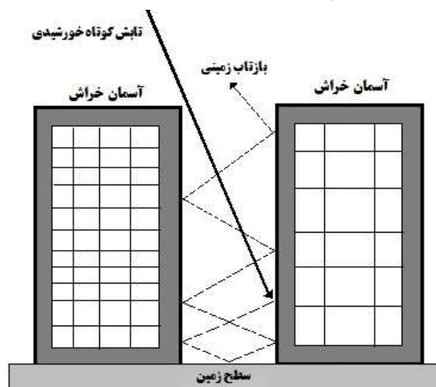
شکل ۷: اثرگذاری ساختمانی در جلوگیری از خروج سریع تابش‌های بلند زمینی
