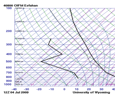
شکل ۳۰. نمودار اسکایوتی ایستگاه اصفهان (الگوی سوم)
