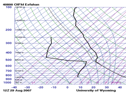
شکل ۲۹. نمودار اسکایوتی ایستگاه اصفهان (الگوی دوم)
