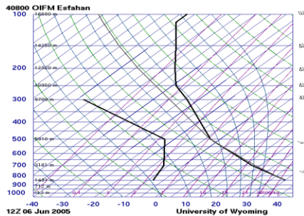
شکل ۳۱. نمودار اسکایوتی ایستگاه اصفهان (الگوی چهارم)
