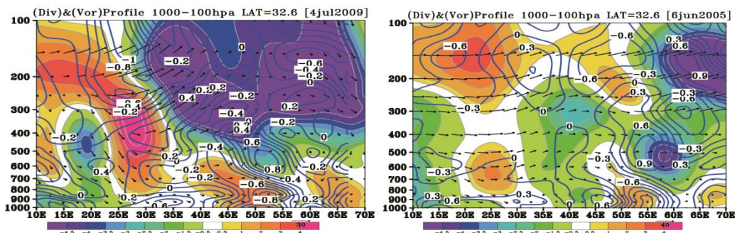
شکل ۱۹. نیمرخ قائم تاوایی و واگرایی برای عرض ۳۲ درجه (عرض شهر اصفهان) (الگوی چهارم)
