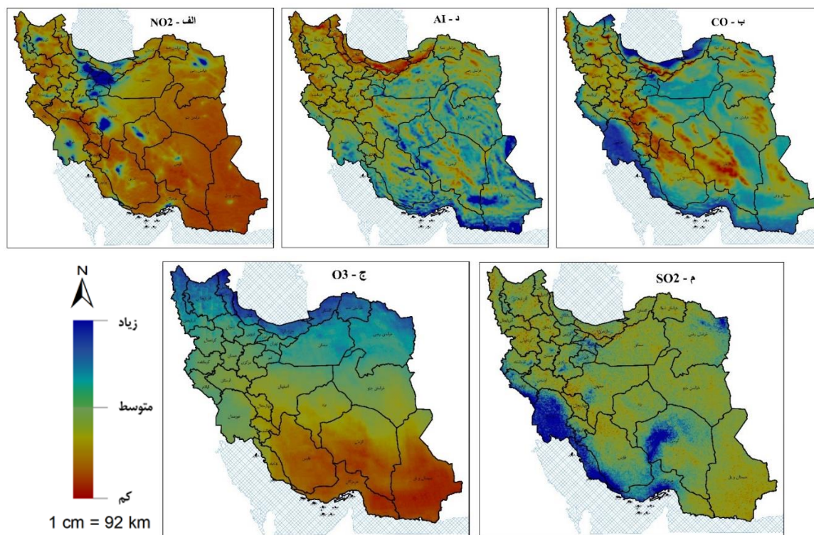
شکل ۸: کانون آلاینده‌های ایران در سال ۱۳۹۸، (الف) \text{NO}_2 ، (ب) \text{CO} ، (ج) \text{O}_3 ، (د) \text{AI} ، (م) \text{SO}_2
