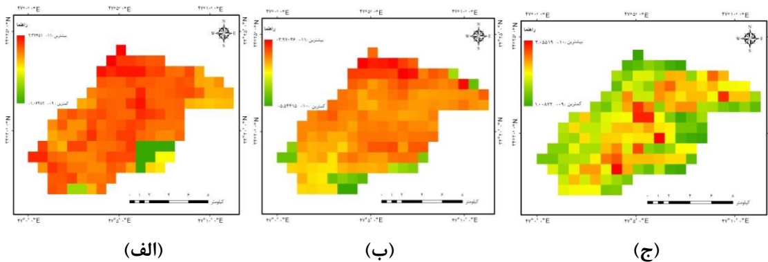
شکل ۱۰: نقشه تغییرات مکانی AOD مربوط به سال‌های (الف): ۲۰۱۶، (ب): ۲۰۱۷ و (ج): ۲۰۱۸ حاصل از تصاویر مودیس
