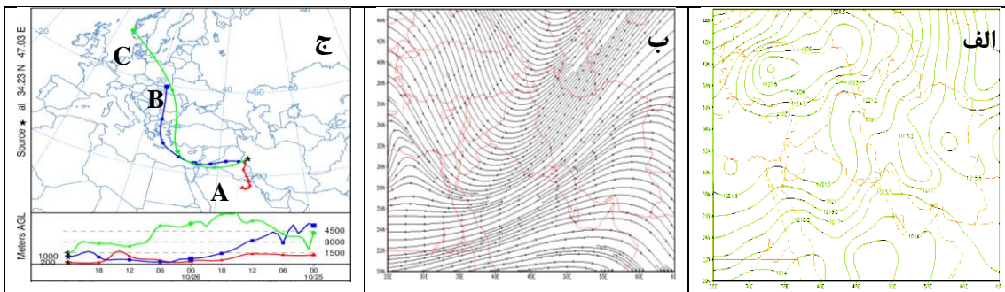
شکل ۶: الف) فشار سطح دریا؛ ب) جریان باد تراز ۳۰۰؛ ج) نقشه ردیابی ذرات گردوغبار HYSPLIT روز ۲۷ اکتبر ۲۰۱۸
