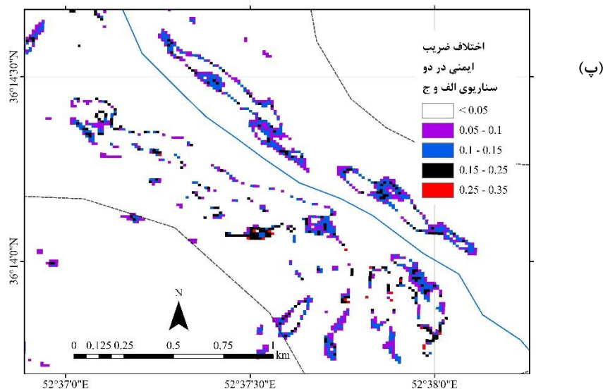
شکل ۱۵- اختلاف ضریب ایمنی حداقل در حوضه آبخیز مورد مطالعه برای شرایط مختلف؛ الف) بعد از گذشت ۶ ساعت از شروع بارش؛ ب) بعد از گذشت ۱۸ ساعت از شروع بارش و پ) نمایش بخشی از نقشه با بزرگنمایی بیشتر (کادر قرمز رنگ در شکل ب) بررسی نقشه‌های ارائه شده در شکل ۱۵ نیز نشان می‌دهد که افت ضریب ایمنی پایداری بعد از وقوع بارندگی‌ها باز هم در بخش‌هایی از زون ۶ که در بخش‌های مرتفع حوضه قرار دارند، بیشتر از نقاط دیگر حوضه رخ داده است. این موضوع نیز با مشاهدات صحرایی همخوانی خوبی نشان می‌دهد، به طوری که بعد از وقوع بارندگی‌های طولانی مدت، ناپایداری‌های دامنه‌ای از نوع لغزش‌های کم‌عمق و جریان گلی-واریزه‌ای در بخش‌های مرتفع حوضه بیشتر از سایر نقاط اتفاق می‌افتند. البته لازم به ذکر است که اینگونه زمین‌لغزش‌ها به دلیل عدم وجود جاده دسترسی مناسب، صعب‌العبور بودن و غیرمسکونی بودن این بخش‌ها، وسعت و عمق کم و عدم اثرگذاری مستقیم بر سکونتگاه‌ها و جاده‌های روستایی منطقه، کمتر شناسایی شده و معمولاً در بانک‌های اطلاعاتی موجود ثبت نمی‌شوند، اگرچه، به دلیل افزایش پتانسیل فرسایش خاک و تأمین مصالح جریان‌های واریزه‌ای می‌توان به طور نسبی آنها را با اهمیت در نظر گرفت. نکته دیگری که از بررسی این نقشه‌ها قابل استنتاج است، این
