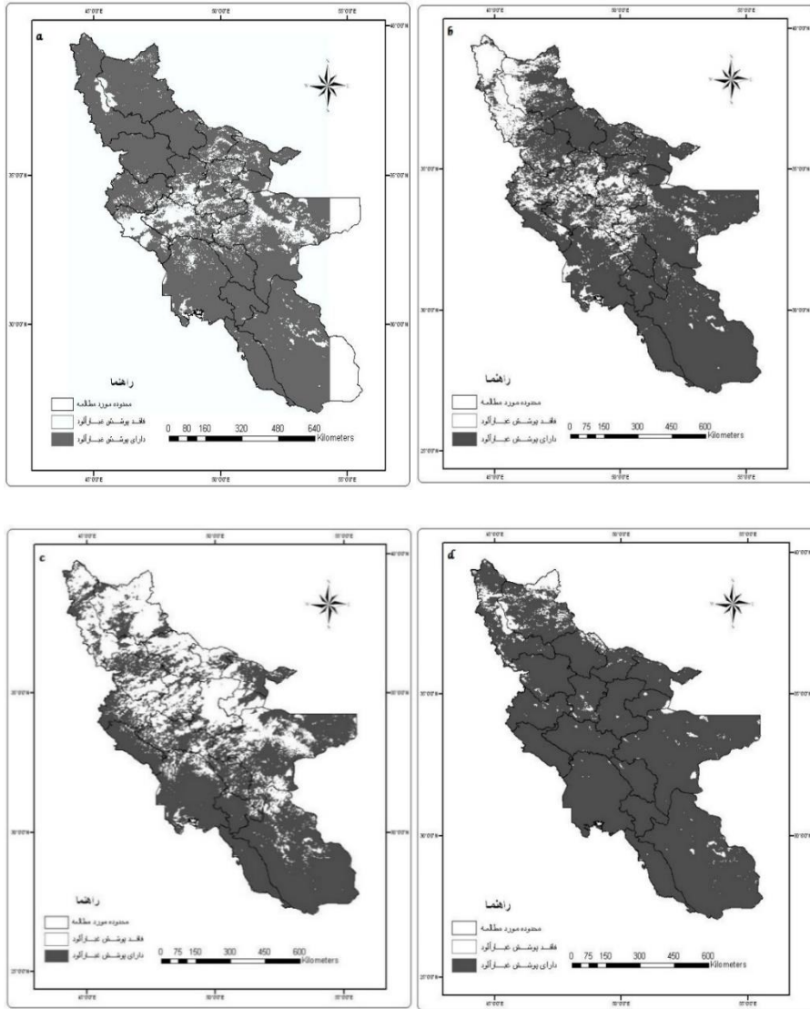
شکل (۵). نقشه‌های نهایی حاصل از بکارگیری شاخص NDDI بر روی تصاویر روزهای (a): اول، (b): دوم، (c): سوم و (d): چهارم جولای ۲۰۰۸
