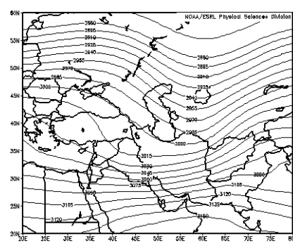
شکل ۱۸. الگوی سینوپتیکی حاکم در تراز ۷۰۰ هکتوپاسکال در روز همراه با بارش برف (الگوی CP۴)
