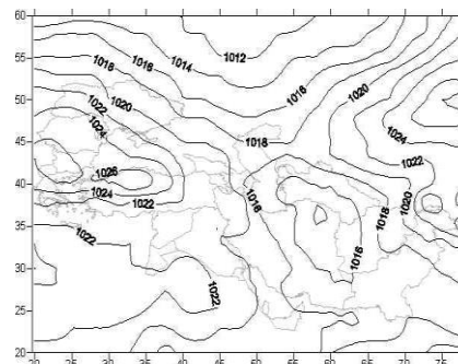
شکل ۲. الگوی سینوپتیکی حاکم در تراز سطح دریا در روز همراه با بارش برف سنگین (الگوی CP 1 )
