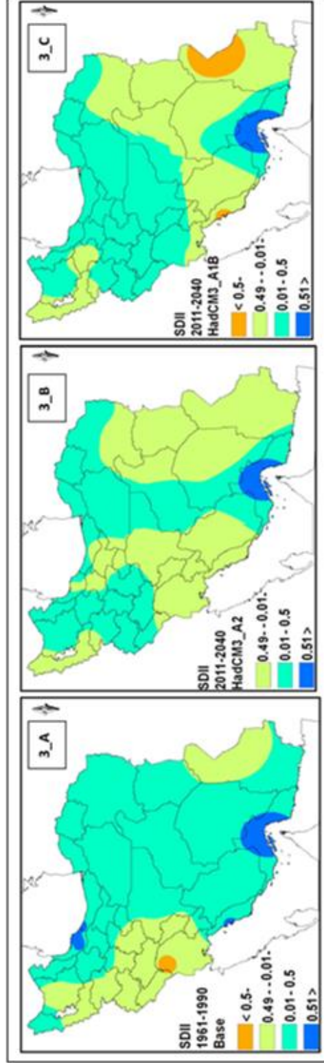
شکل ۳. روند خطی نمایه ساده شدت روزانه بر حسب میزان آن بر دهه طی دوره پایه (۱۹۶۱-۱۹۹۰) و دوره آتی (۲۰۱۱-۲۰۴۰).
