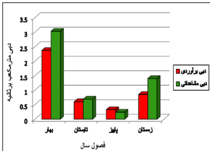
شکل (۱۰). نمودار مقایسه اختلاف دبی برآوردی و مشاهده‌ای حوضه آبخیز افجه
