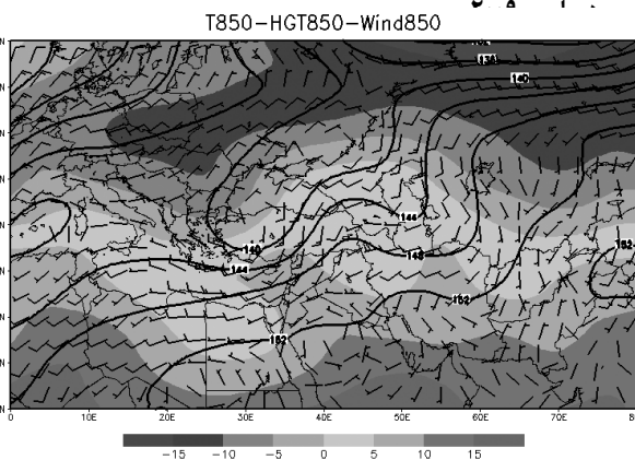
شکل ۱۲: دما (مقادیر رنگی شده بر حسب درجه‌ی سلسیوس)، ارتفاع ژئوپتانسیلی (خطوط هم مقدار بر حسب دکامتر) و میدان باد در تراز ۸۵۰ هکتوپاسکالی برای ساعت ۰۶ گرینویچ روز ۱۳ دسامبر ۲۰۰۹.
