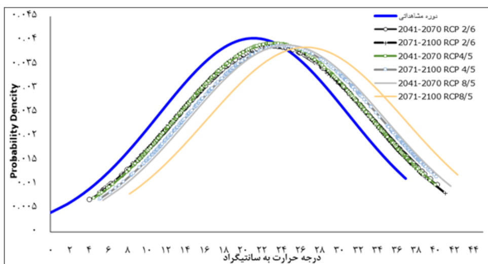
شکل (۵): توزیع حداکثر دمای ماهانه در ایستگاه مشهد نسبت به دوره دیدبانی (۱۹۹۰-۱۹۶۱) در دو دوره ۲۰۴۱-۲۰۷۰ و ۲۰۱۰-
