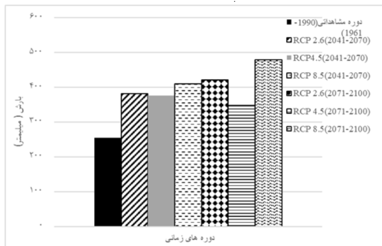
شکل ۲: تغییرات بارش سالانه (میلیمتر) در ایستگاه مشهد در دوره دیدبانی (۱۹۶۱-۱۹۹۰) و دو دوره ۲۰۴۱-۲۰۷۰ و ۲۰۷۱-۲۱۰۰
