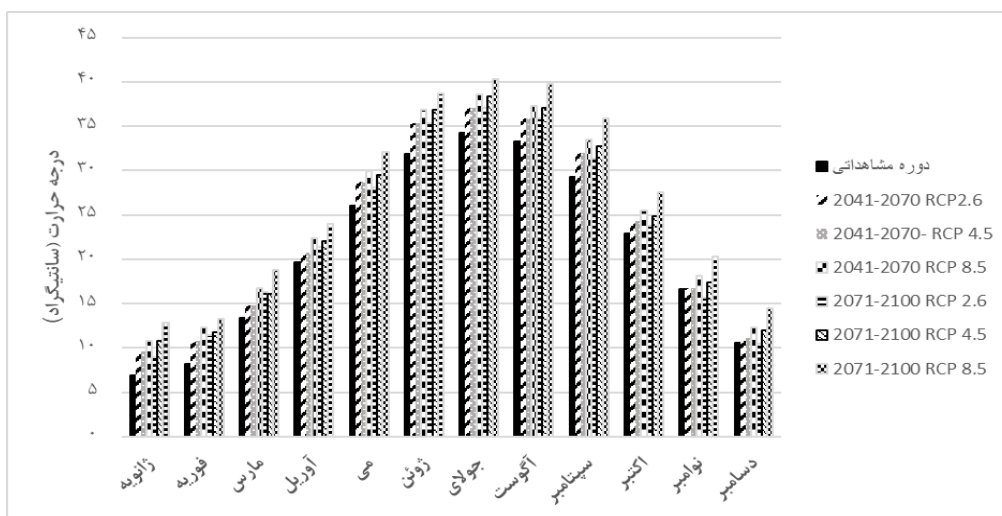
شکل (۴): میانگین دمای حداکثر (سانتی گراد) ماهانه ایستگاه مشهد در دوره دیدبانی (۱۹۹۰-۱۹۶۱) و دو دوره ۲۰۴۱-۲۰۷۰ و
