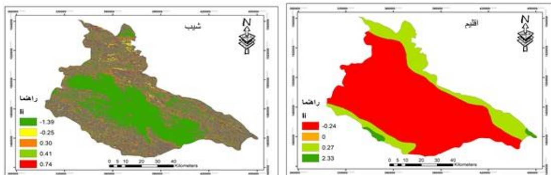
۴) پهنه‌بندی لغزش بر اساس عامل شیب
