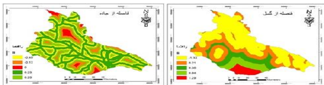
پهنه‌بندی لغزش براساس عامل فاصله از جاده (۱۰)
