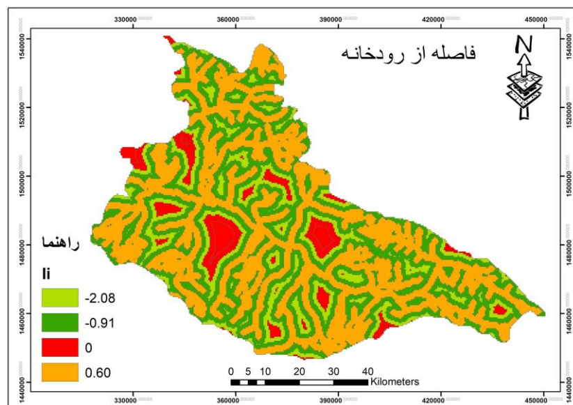
پهنه‌بندی لغزش براساس عامل فاصله از رودخانه (۱۱)
