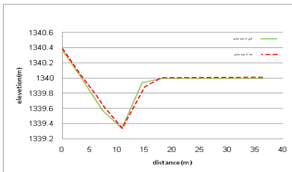
شکل ۴: مقطع عرضی ۱ قبل و بعد از شبیه سازی
