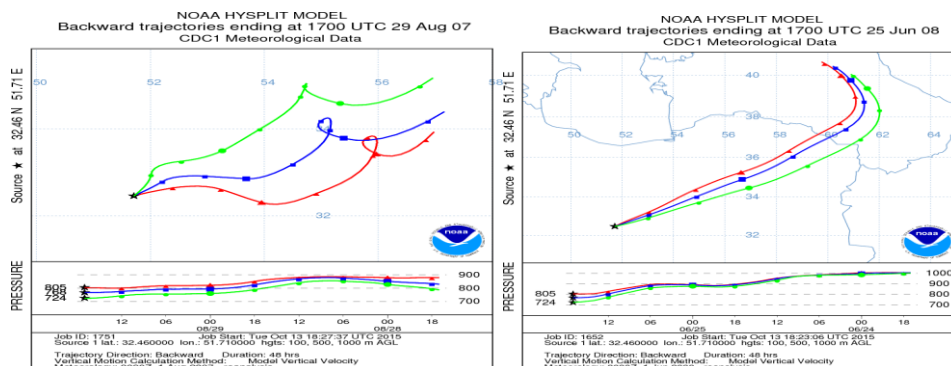
شکل ۲۰. ردیابی ذرات معلق به روش پسگرد (الگوی اول)
