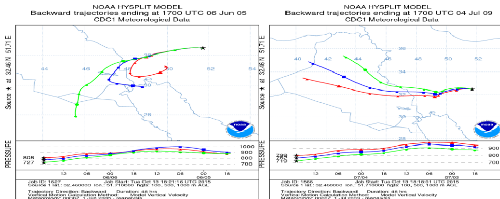
شکل ۲۱. ردیابی ذرات معلق به روش پسگرد (الگوی دوم)
