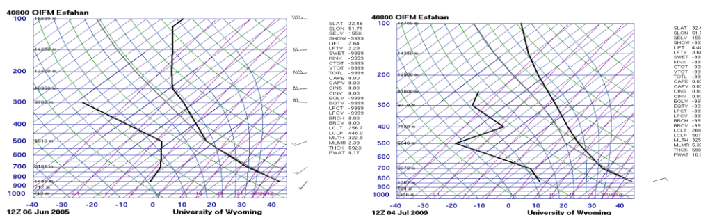
شکل ۳۱. نمودار اسکیتوی ایستگاه اصفهان (الگوی چهارم)
