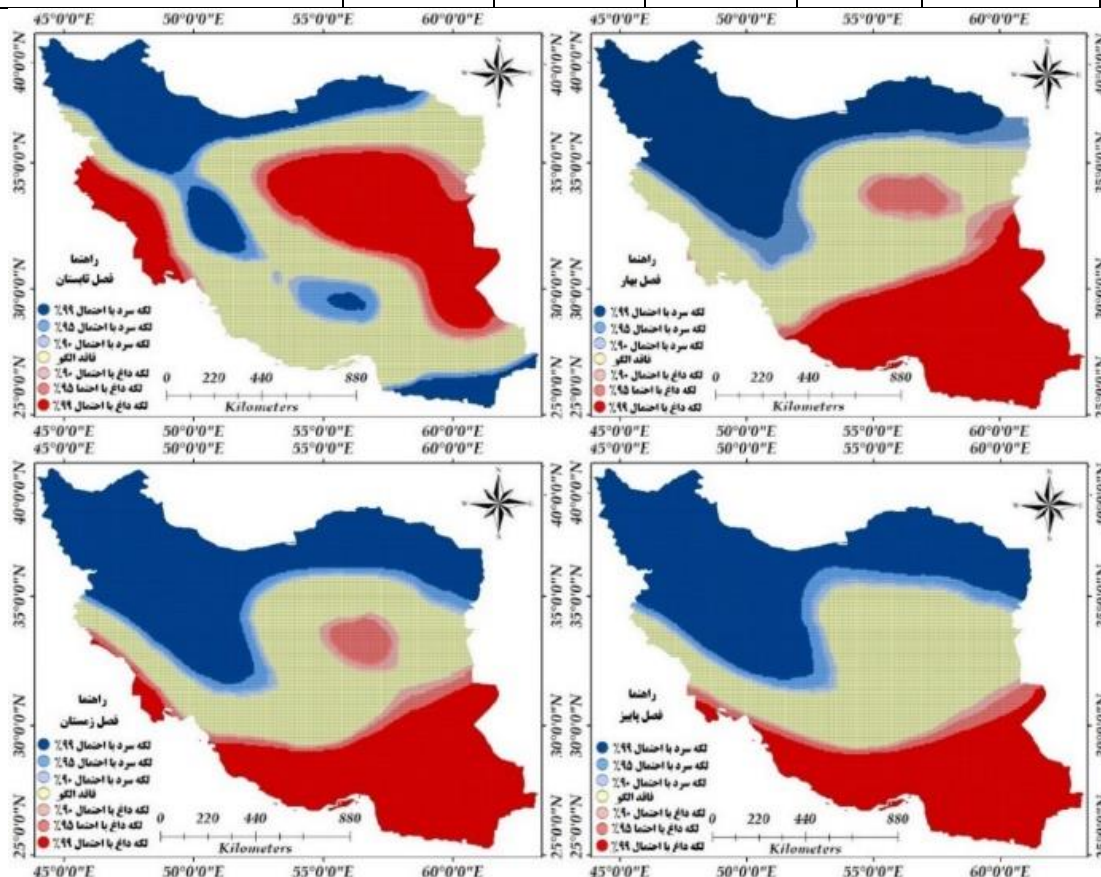
شکل ۷. الگوهای خودهم بستگی فصلی موج بلند خروجی زمین ایران بر اساس شاخص فضایی آماره Gi
