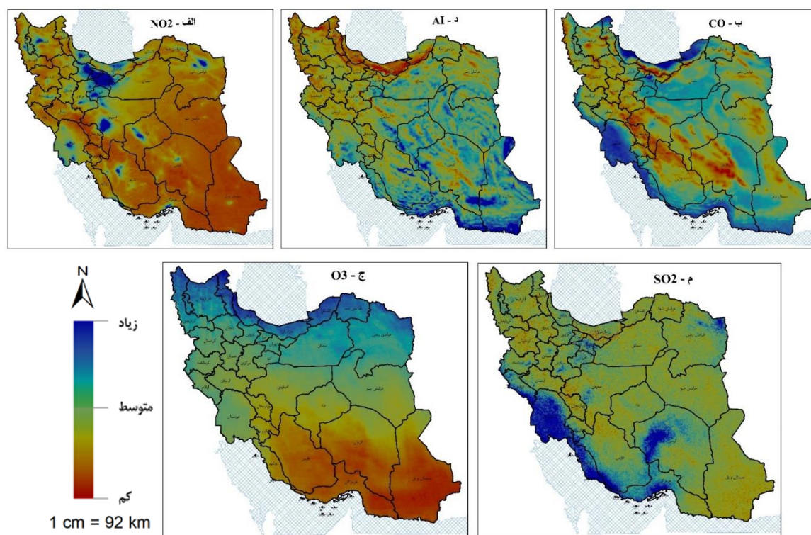
شکل ۸: کانون آلاینده‌های ایران در سال ۱۳۹۸، (الف) NO 2 ، (ب) CO، (ج) O 3 ، (د) AI، (م) SO 2
