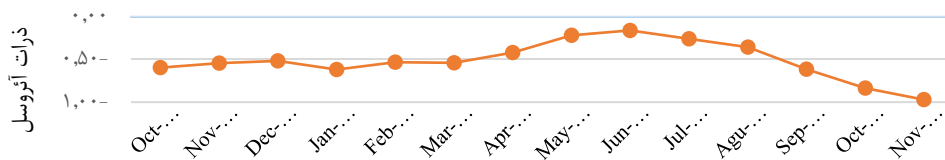
شکل ۵: نمودار تغییرات میانگین ماهانه آلاینده AI در طول ۲۰۱۸-۲۰۱۹
