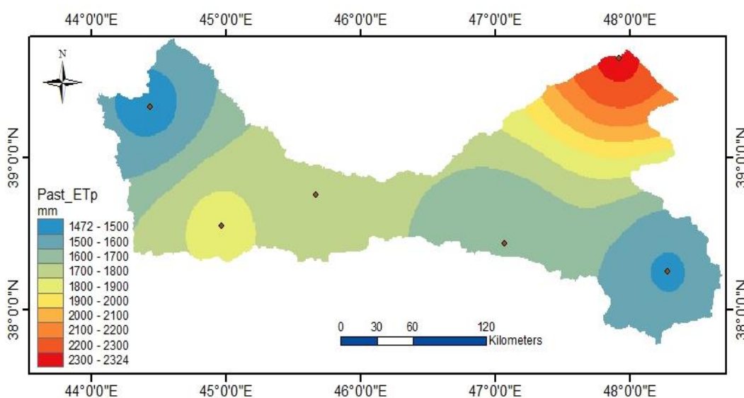
شکل ۴. پراکنش فضایی ETp سالانه حوضه ارس در دوره پایه (۱۹۸۵-۲۰۰۵) بر مبنای داده‌های مدل GFDL
