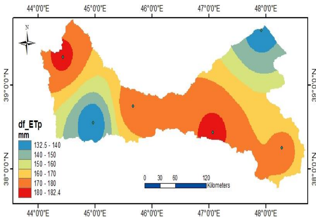
شکل ۶. نقشه تفاضل ET_p آینده (۲۰۲۱-۲۰۵۰) نسبت به گذشته (۱۹۸۵-۲۰۰۵) به روش هارگریوز-سامانی بر مبنای داده‌های مدل GFDL
