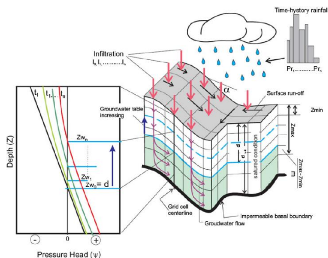
شکل ۷- اجزای مختلف مدل تحلیل پایداری شیب در برنامه ترینگز (Grelle et al., ۲۰۱۴)
