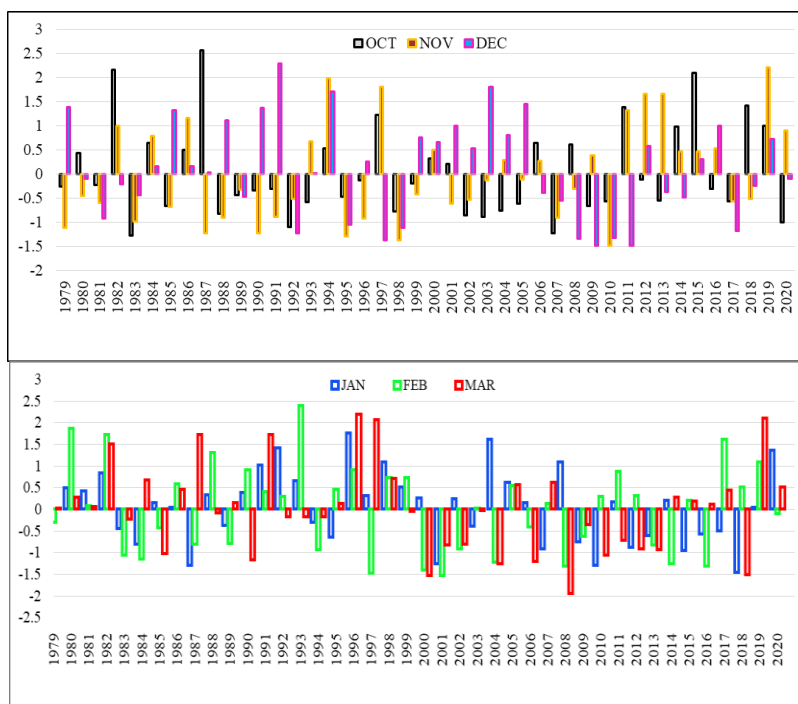
شکل ۲. مقادیر میانگین شاخص SPI جهت شناسایی ماه‌های خشکسالی و ترسالی کشور
