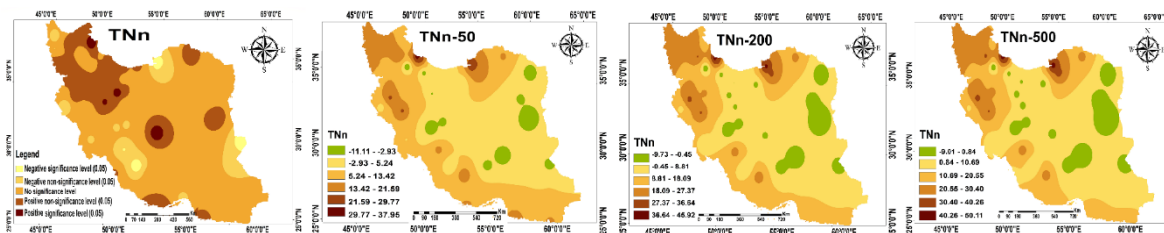
شکل ۹. روند شاخص حدی کمینه دمای حداقل روزانه (TNN) با استفاده از آزمون من-کندال و مقادیر شاخص موردنظر در دوره بازگشت‌های مختلف (اعداد ۵۰، ۲۰۰ و ۵۰۰ بر دوره های بازگشت دلالت دارد).
