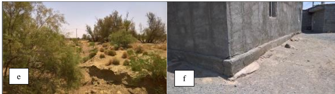
شکل ۱۲: a, b, c و d: شکاف های ناشی از فرونشست زمین و آسیب دیدگی منازل مسکونی در روستای جنگل آباد، e، f: شکاف های ناشی از فرونشست زمین و آسیب دیدگی منازل مسکونی در روستای چراغ آباد
