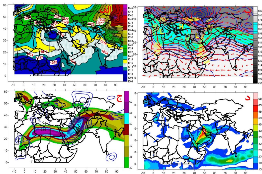
شکل ۸. الف) فشار سطح دریا به پاسکال ب) ارتفاع ژئوپتانسیل تراز ۵۰۰ هکتوپاسکال به متر و جهت جریان باد تراز ۵۰۰ هکتوپاسکال به متر بر ثانیه ج) امگا تراز ۵۰۰ به پاسکال و رودباد تراز ۲۵۰ هکتوپاسکال به متر بر ثانیه د) رودخانه جوی کیلوگرم متر بر ثانیه
