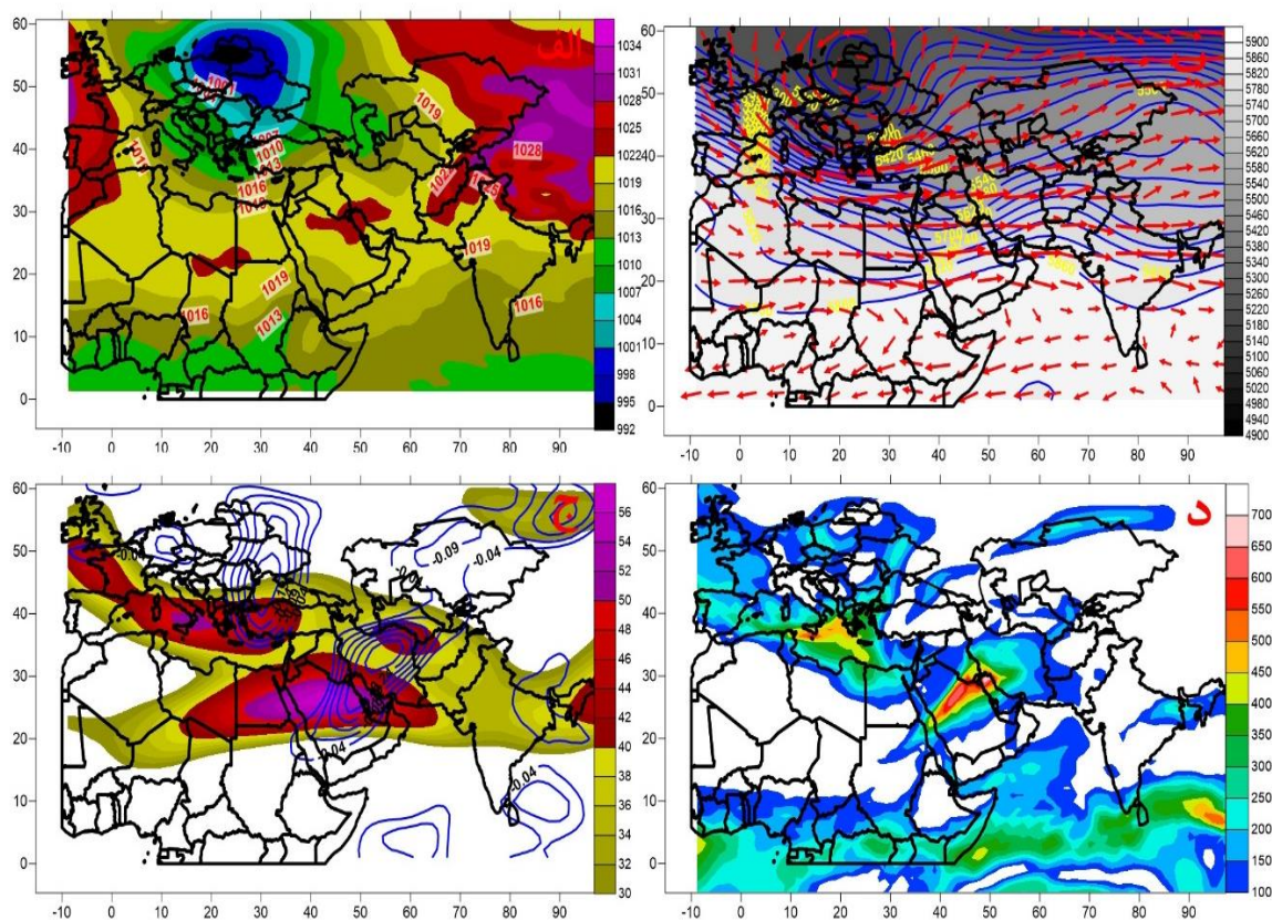
شکل ۷. الف) فشار سطح دریا به پاسکال ب) ارتفاع ژئوپتانسیل تراز ۵۰۰ هکتوپاسکال به متر و جهت جریان باد تراز ۵۰۰ هکتوپاسکال به متر بر ثانیه ج) امگا تراز ۵۰۰ به پاسکال و رودباد تراز ۲۵۰ هکتوپاسکال به متر بر ثانیه د) رودخانه جوی کیلوگرم متر بر ثانیه
