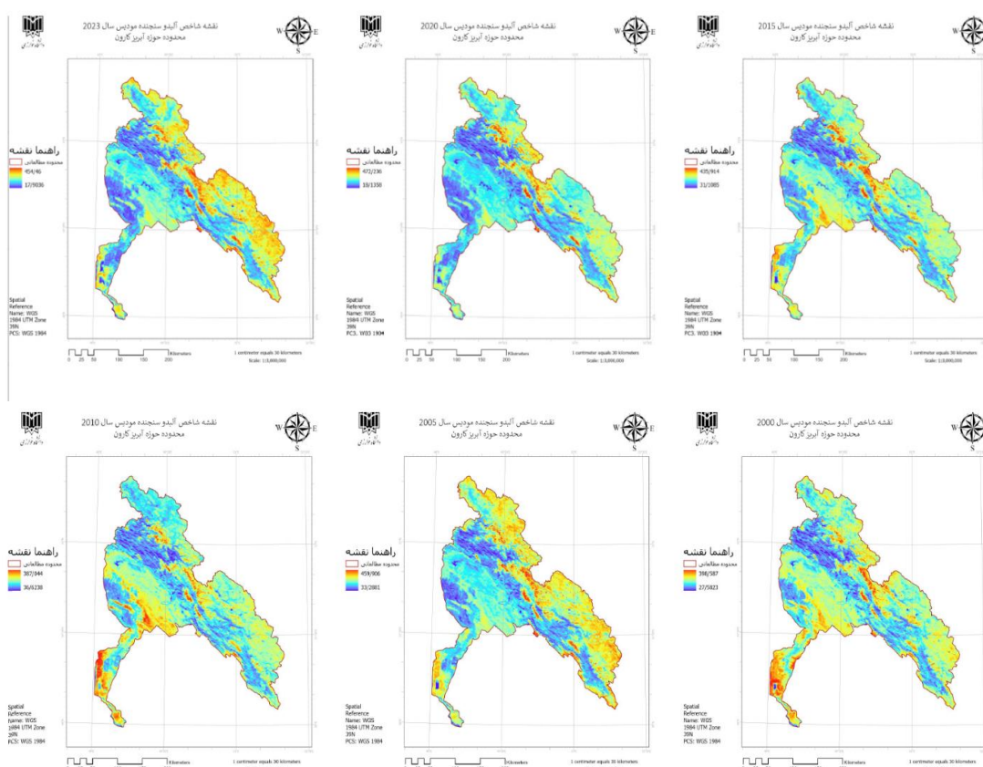
شکل ۲۰. نقشه های شاخص آلبدو حوزه آبریز کارون، میانگین سالانه ۲۰۰۰ تا ۲۰۲۳
