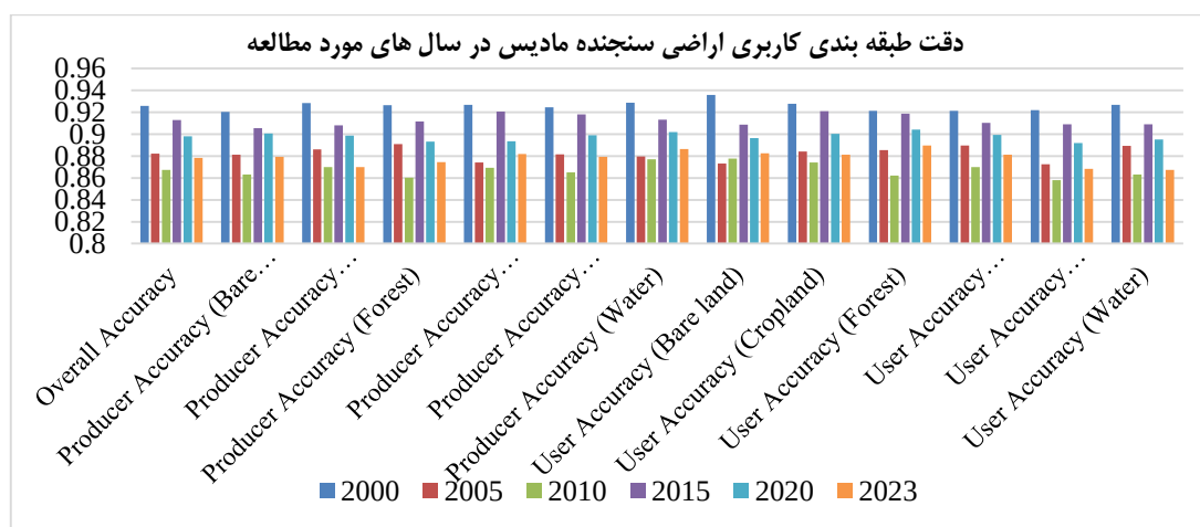
شکل ۶. نمودار دقت طبقه بندی کاربری اراضی سنجنده مادیس در سال های ۲۰۰۰ تا ۲۰۲۳
