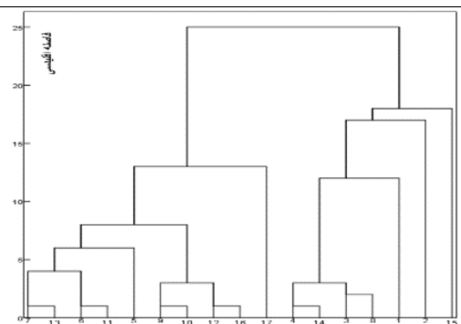
شکل ۵. بارش های مربوط به خوشه ۳
