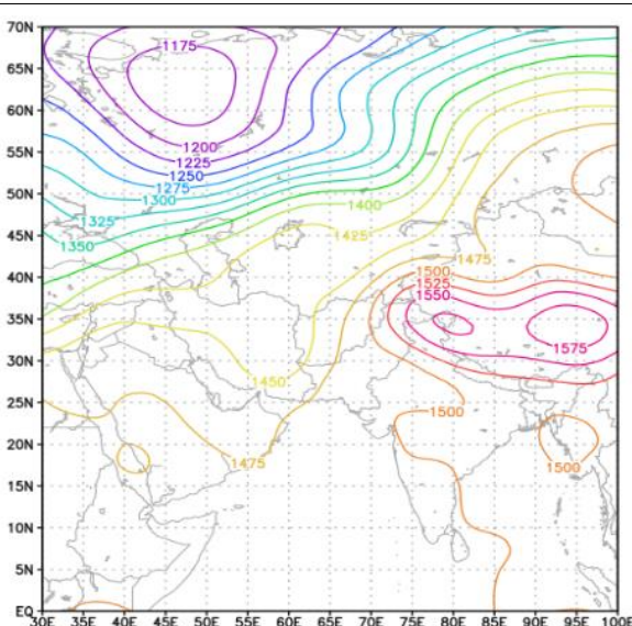
شکل ۹. نقشه تراز ۸۵۰ هکتوپاسکال تاریخ ۲۳ مارس ۲۰۰۹ (ساعت ۰۰ UTC)
