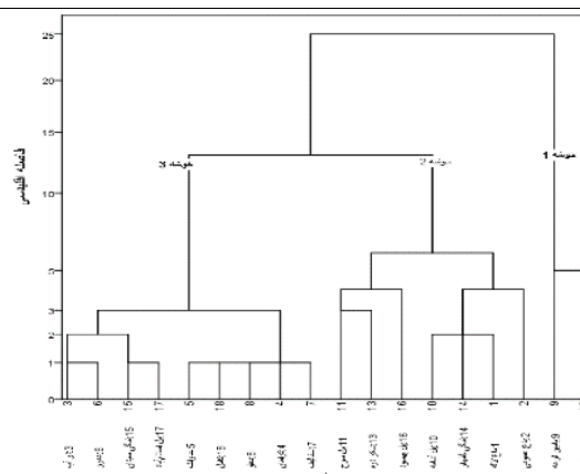
شکل ۲. نمودار درختی روز های بارشی برای بارش های بالاتر از ۲۰ میلی متر
