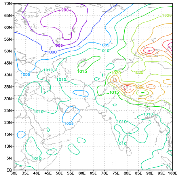
شکل ۷. نقشه تراز دریا تاریخ ۲۳ مارس ۲۰۰۹ (ساعت ۰۰ UTC)
