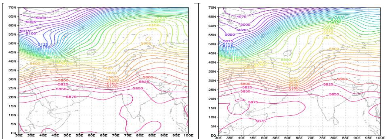
شکل ۲۳. نقشه‌ی تراز ۵۰۰ هکتوپاسکال روز ۱۷ مارس ۲۰۱۴ (ساعت ۱۲ UTC)
