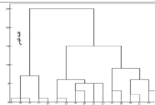
شکل ۴. بارش های مربوط به خوشه ۲
