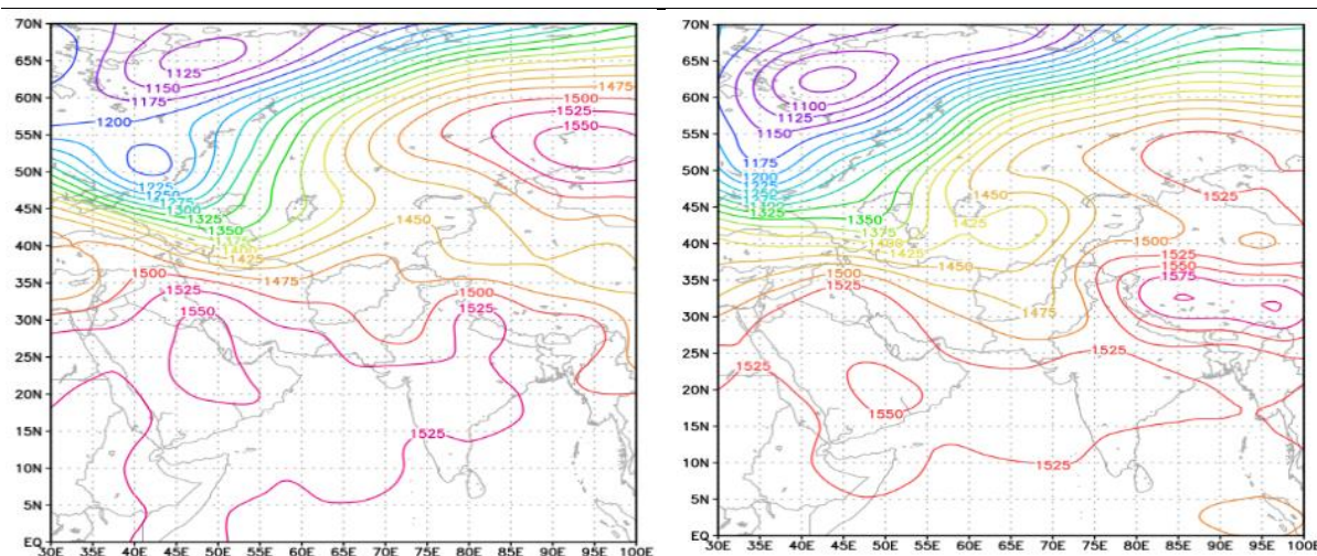
شکل ۲۱. نقشه‌ی تراز ۸۵۰ هکتوپاسکال روز ۱۷ مارس ۲۰۱۴ (ساعت ۱۲ UTC)
