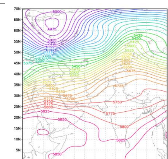
شکل ۱۱. نقشه تراز ۵۰۰ هکتوپاسکال تاریخ ۲۳ مارس ۲۰۰۹ (ساعت ۰۰ UTC)
