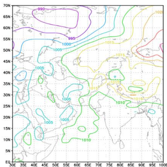
شکل ۸. نقشه تراز دریا تاریخ ۲۳ مارس ۲۰۰۹ (ساعت ۱۲ UTC)
