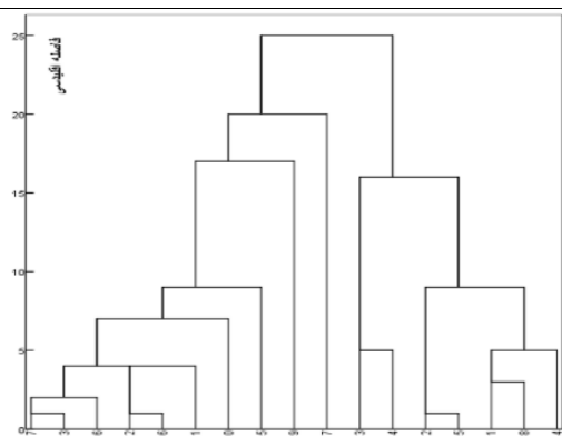
شکل ۳. بارش مربوط به خوشه ۱
