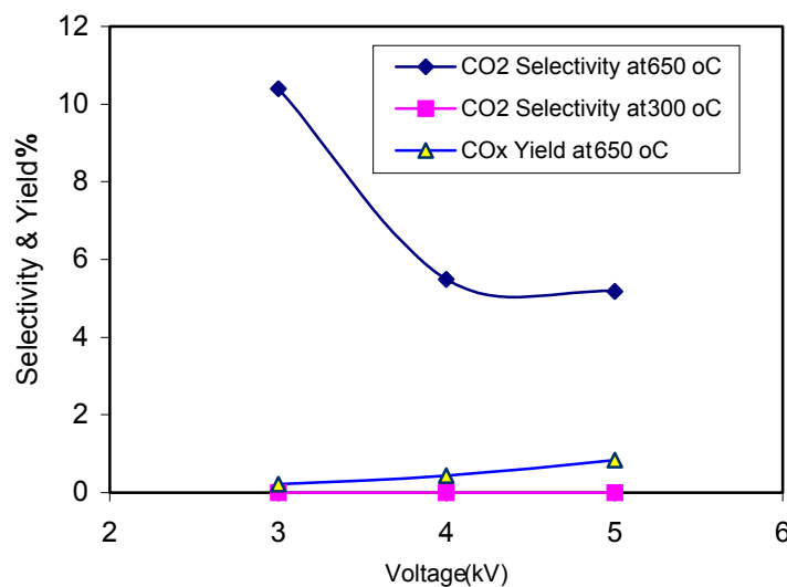
شکل ۱۲ - تاثیر ولتاژ برگزینش‌پذیری و راندمان نهایی محصول به گاز کربنیک در دماهای ۶۵۰ و ۳۰۰ درجه سانتی‌گراد در \text{CH}_4/\text{O}_2 = 4/1
