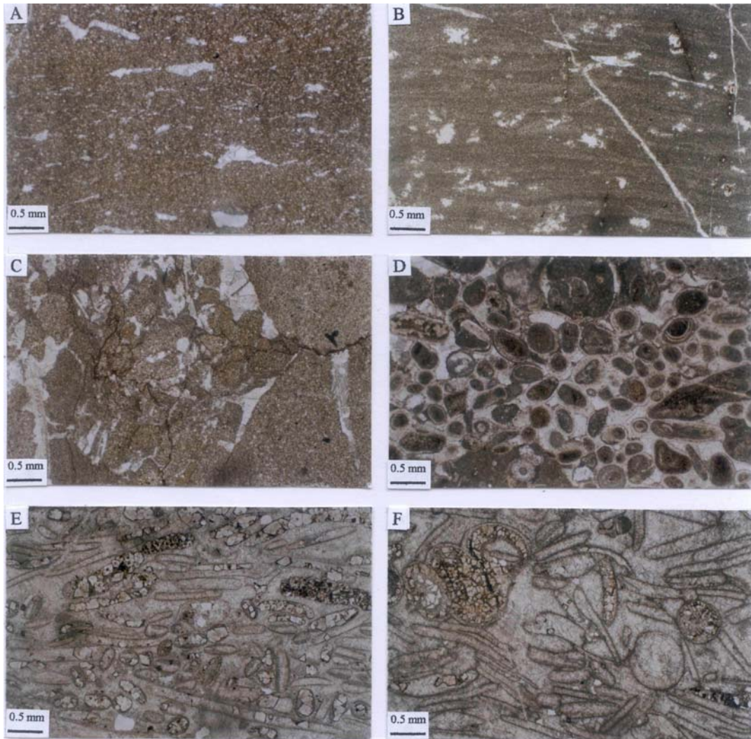
شکل ۴- A- دولومدستون با فابریک چشم پرنده‌ای مربوط به رخساره C ، مقطع توسط الیزارین قرمز رنگ‌آمیزی شده است (نمونه برش گذار سرخ) B- دولومدستون لامینه‌دار با فابریک چشم پرنده‌ای و قالب‌های دروغین ژپیس و انیدریت در رخساره C، مقطع توسط الیزارین قرمز رنگ‌آمیزی شده است (نمونه از برش اسلام‌آباد) C- گرینستون اینتراکلاستی از رخساره طوفانی کریناته، در این تصویر، اینترکلاست‌های میکریتی بوده‌اند و فابریک سیمان از نوع هم بعد است. بالای مقطع به سمت چپ عکس است بنابراین ساختمان رسوبی از نوع لایه‌بندی تدریجی نیز در اینجا مشاهده می‌گردد (نمونه از برش گذار سرخ) D- گرینستون الیدی اینتراکلاستی مربوط به رخساره طوفانی کریناته. الیدها دارای فابریک‌های شعاعی و متحد‌المركز هستند. فابریک سیمان نیز غالباً از نوع هم بعد است (نمونه از برش گذار سرخ) E- گرینستون بیوکلاستی الیدی از رخساره طوفانی کریناته. الیدها دارای فابریک متحد‌المركز بوده و دوکفه‌ای‌ها نیز توسط کلسیت اسپاری پر شده‌اند. فابریک‌های سیمان از نوع دروزی موزائیکی و هم قعد هستند بلورهای اتومورف دولومیت نیز به وضوح دیده می‌شوند. برخی از آنها حالت زونه مانند نیز دارند (نمونه از برش گذار گچال) F- گرینستون بیوکلاستی در رخساره طوفانی کریناته. بیوکلاست‌ها شامل دوکفه‌ای و شکم‌پایا دیواره اسپاریتی هستند. فابریک‌های سیمان از نوع هم بعد و دروزی موزائیکی‌اند جانشینی بلورهای اتومورف دولومیت در برخی از آوکه‌ها دیده می‌شوند (نمونه از برش گذار گچال)
