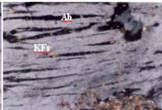
شکل ۸. نمایش بافت پرتیت (هم‌رشدی آلبيت و فلدسپات پتاسیک) در توده گرانیتی شمال موته ( \times 100.XPL ). فلدسپات پتاسیک = Kfs و آلبيت = Ab
