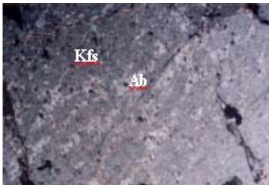
شکل ۹. هم‌رشدی‌های پرتیتی (سرد شدن و اختلاط ناپذیری) در گرانیت‌های شمال موته ( \times 100.XPL ). فلدسپات پتاسیک = Kfs و آلبيت = Ab
