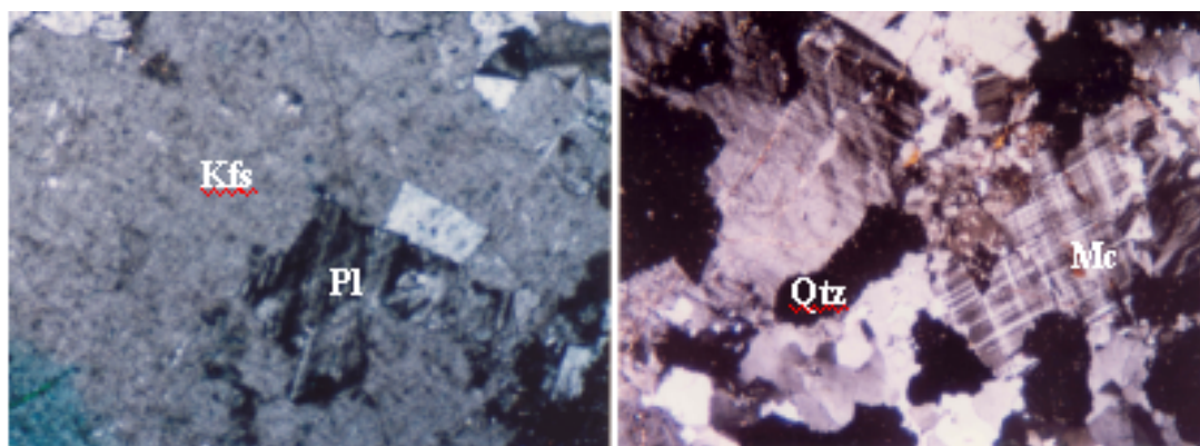
شکل ۵. تصویر بافت بوئی کلینی که در آن فلدسپات پتاسیک پلاژیوکلاز را در بر گرفته است (×100.XPL) فلدسپات پتاسیک = Kfs و پلاژیوکلاز = Pl
