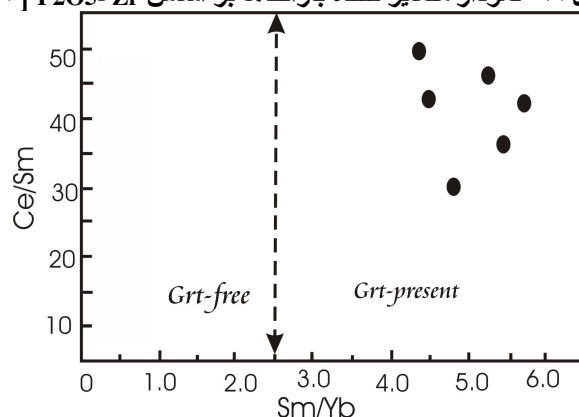
شکل ۱۴- موقعیت سنگ‌های آتشفشانی منطقه جهق در نمودار Ce/Sm در برابر Sm/Yb، (اقتباس از [۱۴])
