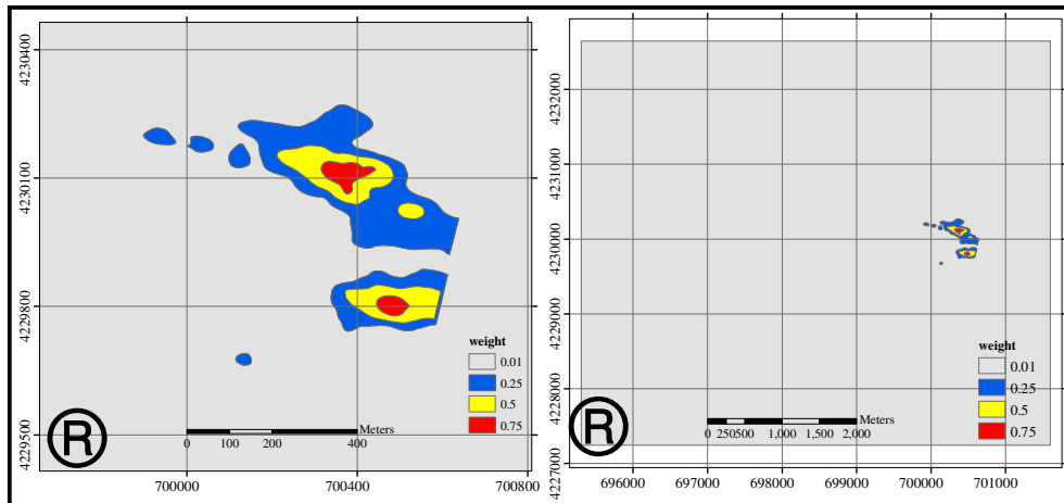
شکل ۸. نقشه فاکتور شارژ ایلیتیة
