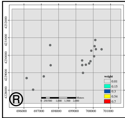
شکل ۴. نقشه فاکتور نشانه های کانی سازی
