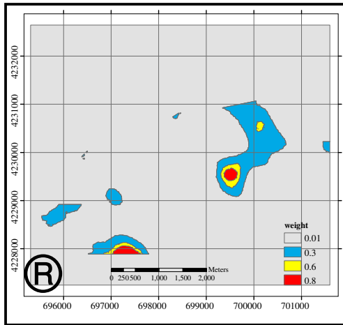
شکل ۵. نقشه فاکتور عیار مس
