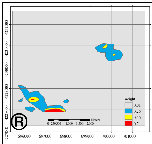
شکل ۷. نقشه فاکتور عیار طلا
