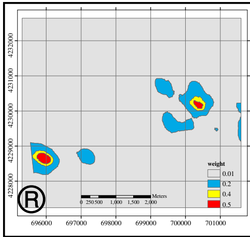
شکل ۶. نقشه فاکتور عیار مولیبدن
