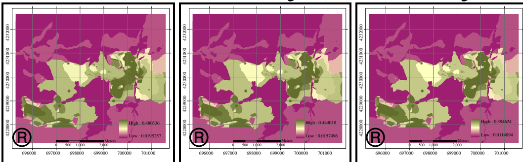
شکل ۱۶ - نقشه پتانسیل معدنی عملگر عملگر فازی \Gamma = 0.97
