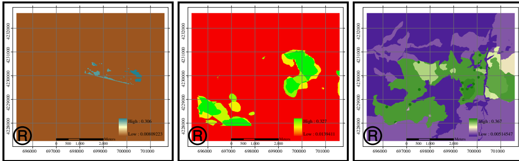
شکل ۱۳ - نقشه پتانسیل معدنی ژئوفیزیک Sum
