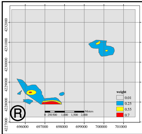
شکل ۷. نقشه فاکتور عیار طلا
