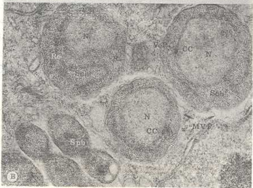
شکل ۳ - باکوله آدافنیه: شیزونت با هسته‌های در شروع تقسیم. 60000 \times A و 33000 \times B . ریپوزوها = R ، هسته = N ، غشا واکوئل انگلی = MVP ، غشا پلاسمیک = MP ، مرکز جنبشی = CC کیسه‌های قطبی شده = VeP ، سپرو بلاست = Spb ، شیزونت = Sch ، شبکه داخل سینوپلاسمی = Re
