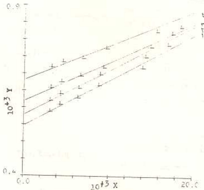
شکل ۳ - نمایش تغییرات y = 10^3 C_{VO_2} / A بر حسب x = 10^3 (A - \epsilon_0 C_{VO_2}) [H]^+ / A در طول موجهای (۱) ۲۶۰، (۲) ۲۶۵، (۳) ۲۷۰، (۴) ۲۷۵ نانومتر و در دمای ۳۰°C.
