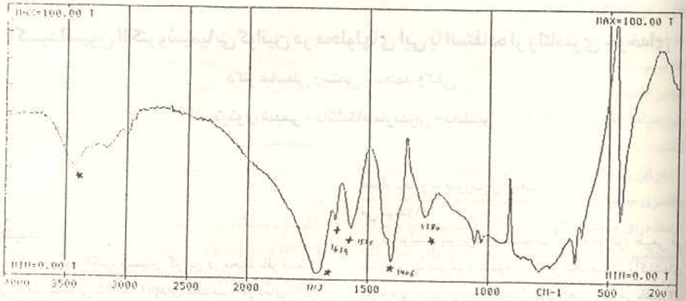
شکل ۱: طیف IR از نمک سدیم هیدروژن استات.
